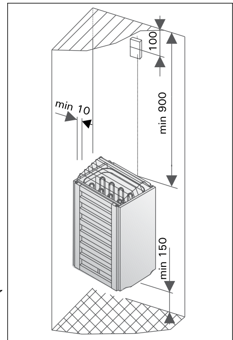
Figure 13. Installation of the sensor of C90 control unit Abbildung 13. Installation des Fühlers des Steuergerätes C90
