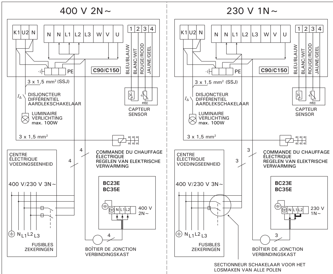
Figure 11. Centre de contrôle C90/C150 et raccords électriques du poêle BC-E Figuur 11. Elektrische aansluitingen van de besturingsunit C90/C150 en saunaoven BC-E
